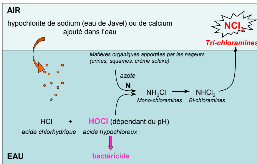
Figure 1 : Formation de dérivés volatiles azotés (d'après réf. 9)
